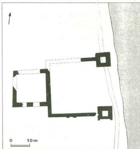
A Dera-patak torkolatánál, Szentendre déli határában fekvő későrómai hídfoállítás alaprajza
